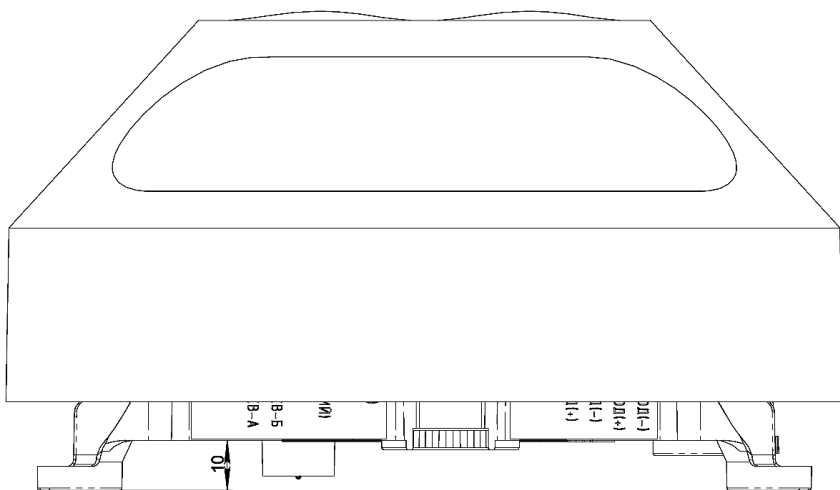
Рисунок 3 – Пространство для кабелей под основанием блока ППРД
